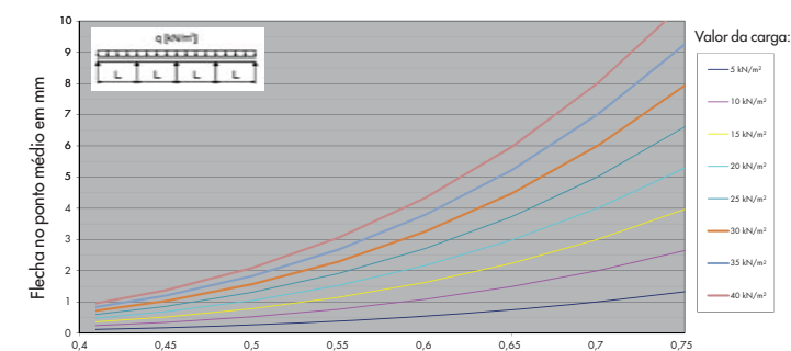
Flecha do painel de três camadas de 21mm
