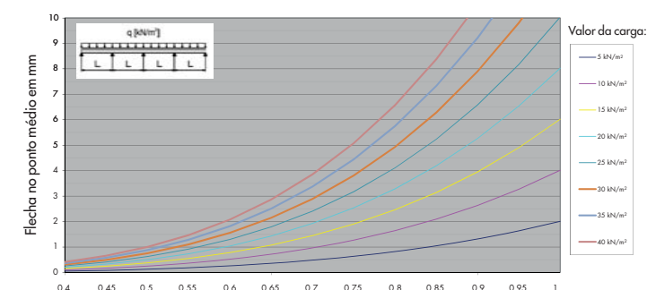
Flecha do painel de três camadas de 27mm
